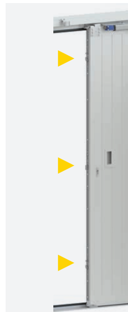
Serrure 3 points
