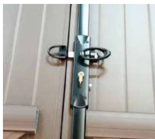
Serrure 3 points de série
